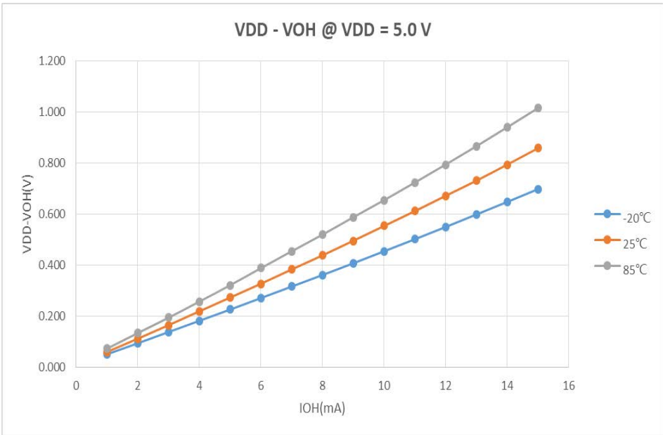
Figure 3-1 ( V_{DD}-V_{OH} ) 温度曲线
